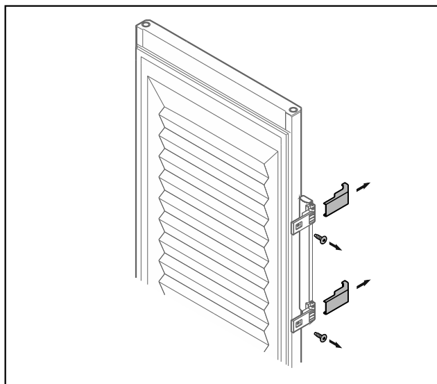
Fig. 24 Geschuimde deur*
