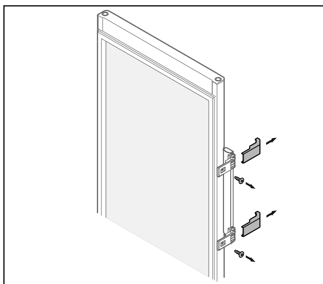
Fig. 25 Glasdeur*
