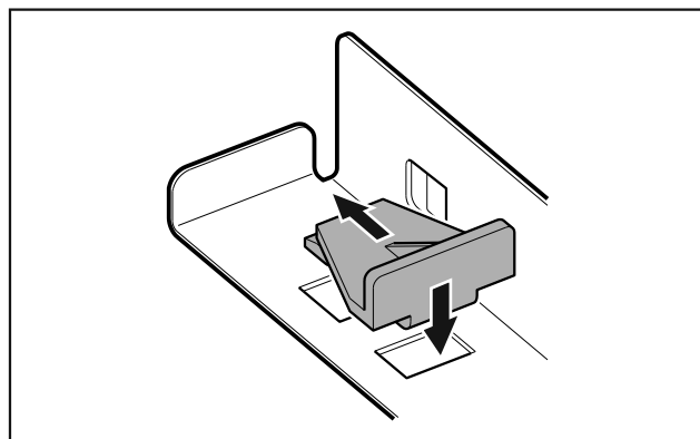
Fig. 55 Stophoek plaatsen
